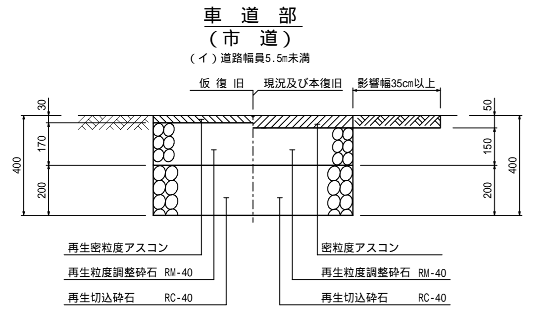
舗装構造図 縮尺 1:15
