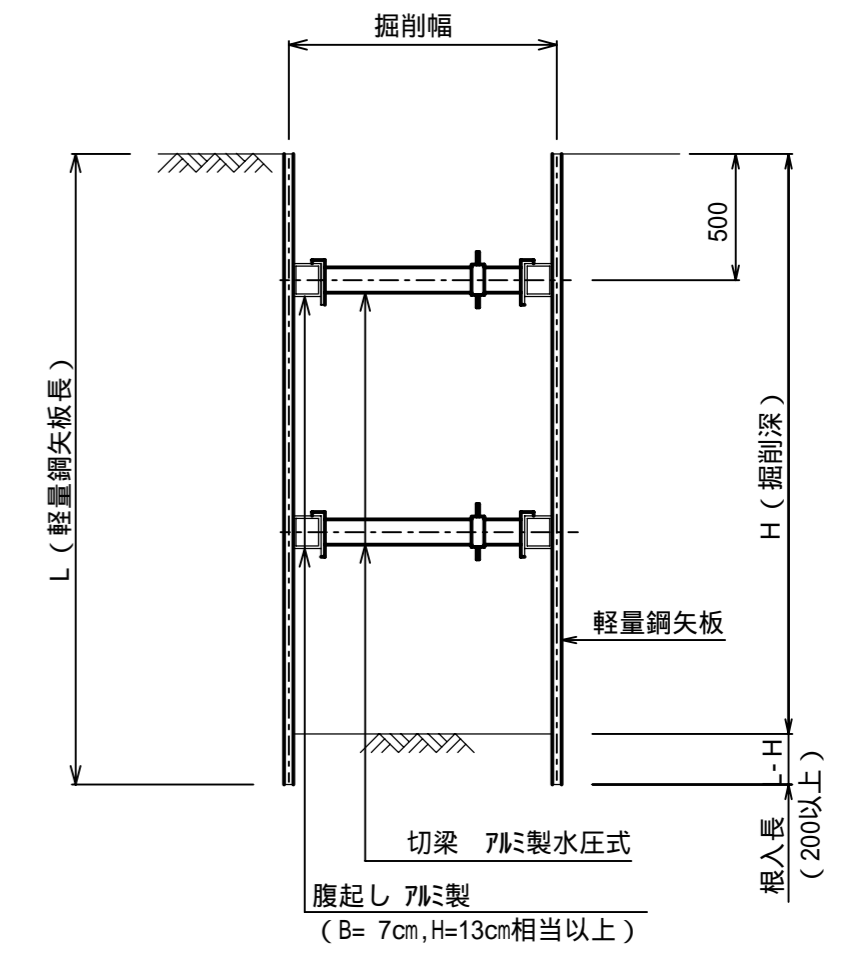
軽量鋼矢板 L=3.00m (掘削深 2.3m以上2.8m未満)
