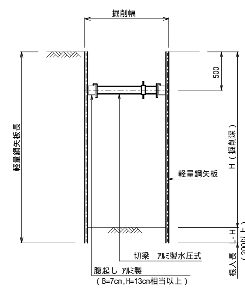
軽量鋼矢板 L=2.50m (掘削深 1.8m以上2.3m未満)
