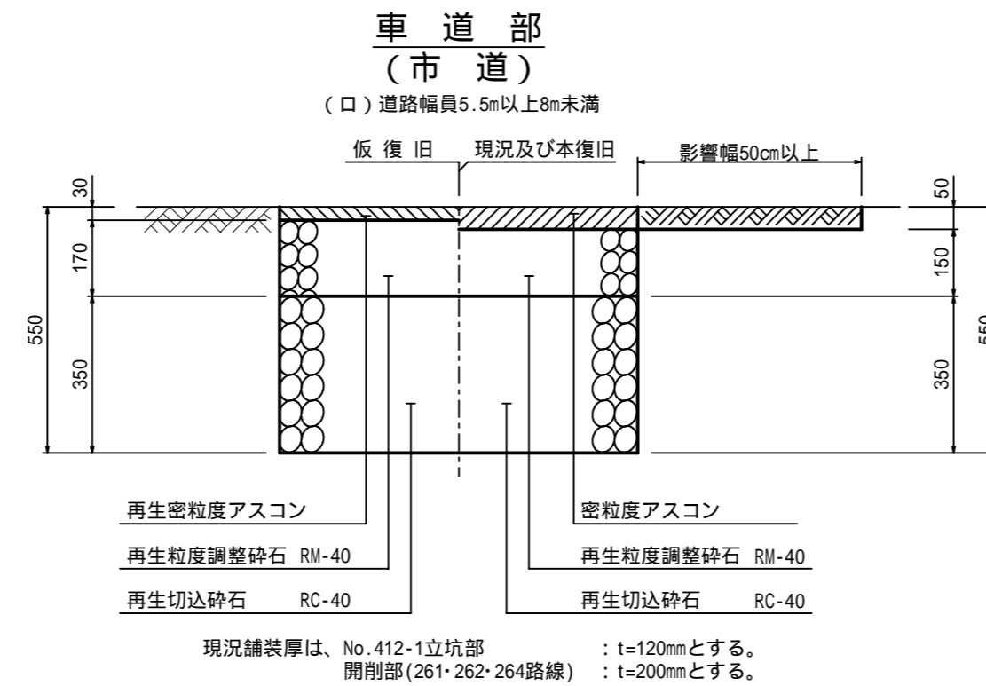
舗装構造図 縮尺 1:15
